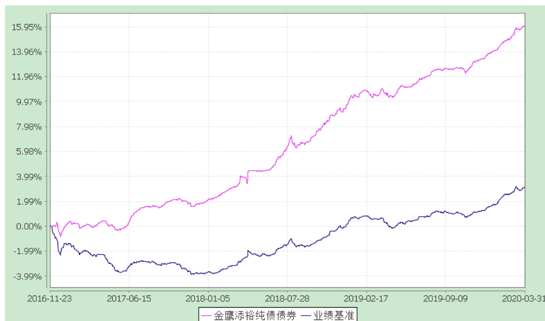
金鹰添裕纯债债券型证券投资基金 累计净值增长率与业绩比较基准收益率历史走势对比图 (2016 年 11 月 23 日至 2020 年 3 月 31 日)
